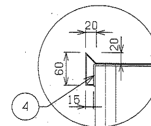
A部詳細
