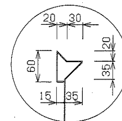
A部詳細
